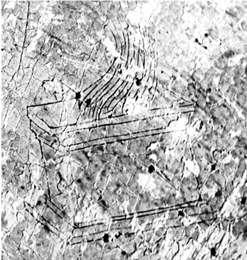
Cusanus globe
