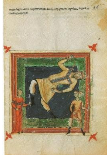
Jupiter – detriment
